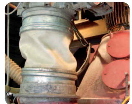
staubfreie BFM®-Muffe
